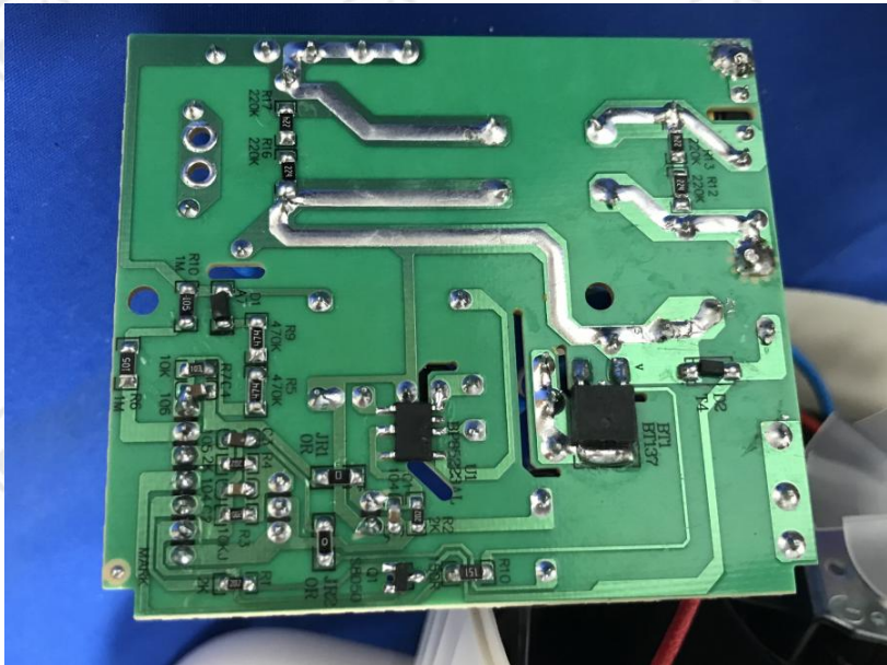
Fig.10- Main PCB
